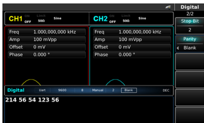
Рис. 147 Установка стопового бита
