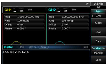
Рис. 184 Установка ручной отправки данных
