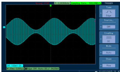
Рис. 26 Осциллограмма сформированного амплитудно-модулированного сигнала
