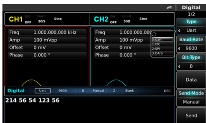
Рис. 149 Выбор функции UART
