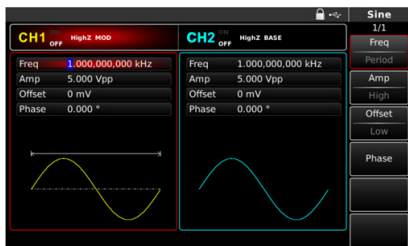
Рис. 90 Установка частот несущего сигнала
