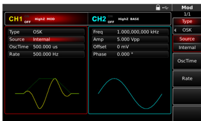
Рис. 84 Установка частот несущего сигнала
