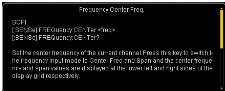
Рис. 1-14 Справочный интерфейс
