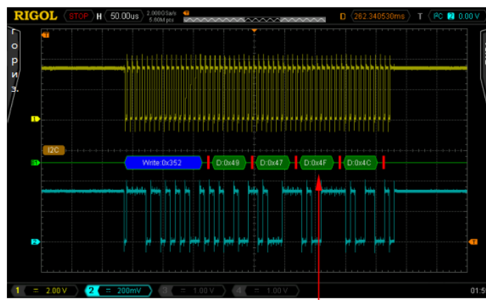
ACK=1
