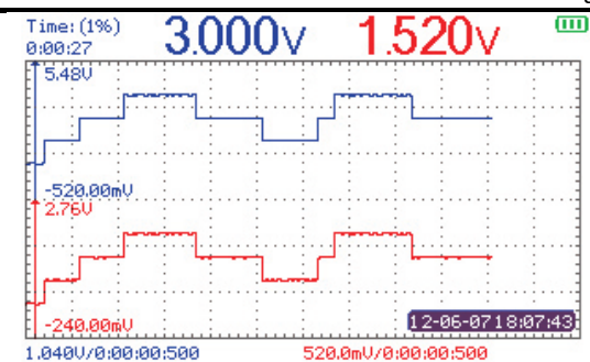
Экран регистратора (TREND PLOT в режиме Осциллограф)
